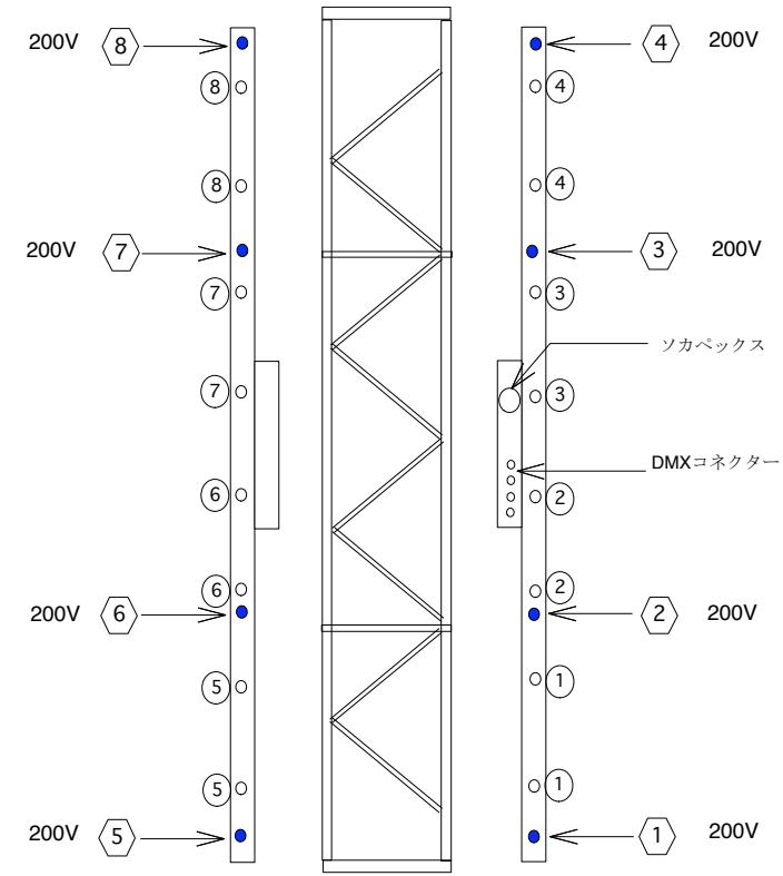
SHIBUYA AX サイドトラス回路図
